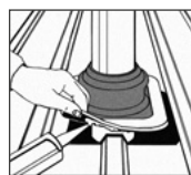
3. Dichtungsmasse auftragen.
