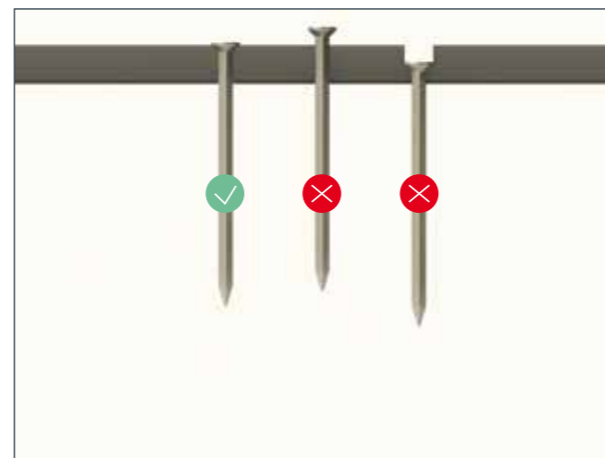
Befestigungen nicht versenken oder abwinkeln. Die Befestigungen müssen bündig mit der Oberfläche der Cembrit Plank abschließen.
