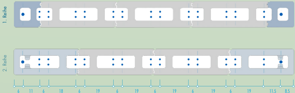
Gerade Mauer mit 17,5 cm Wandstärke
