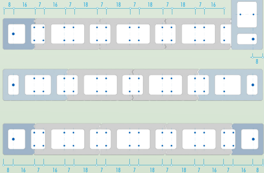
Gerade Mauer mit 24 cm Wandstärke
