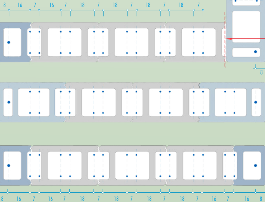
Gerade Mauer mit 30 cm Wandstärke
