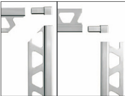
Schlüter®-QUADEC Außen- und Innenecken
