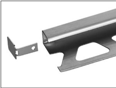
Schlüter®-QUADEC-EB/EK (Endkappe Edelstahl gebürstet für QUADEC-E und -EB)
