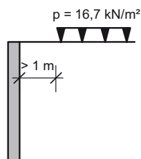
Lastfall 16,7 kN/m 2
