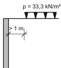
Lastfall 33,3 kN/m 2
